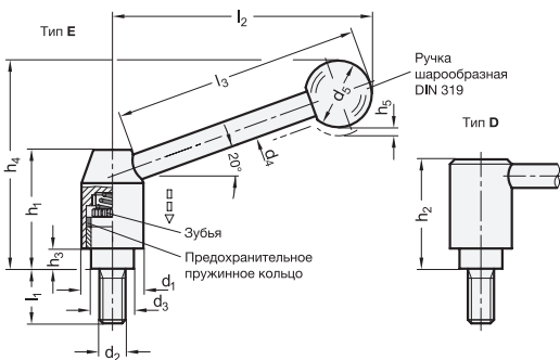
GN 312-с резьбовым стержнем
